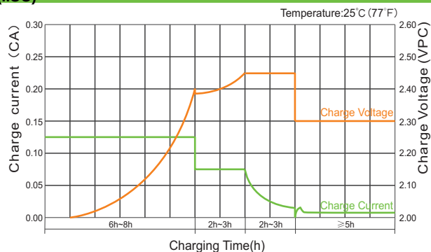
Courbe caractéristique de charge pour l'utilisation du cycle (IUIU)
