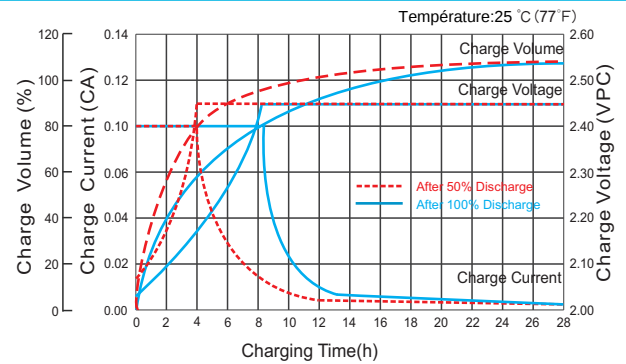
Courbe de charge caractéristique pour utilisation cyclique(IU)
