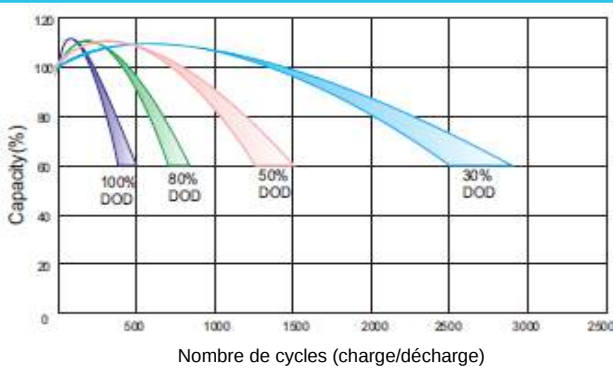
Caractéristiques du cycle de vie utile
