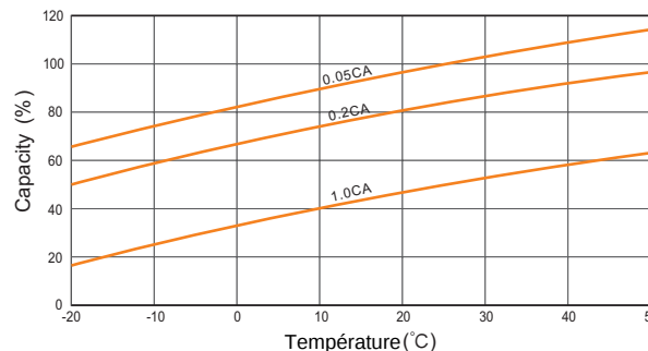
Effets de la température sur la capacité
