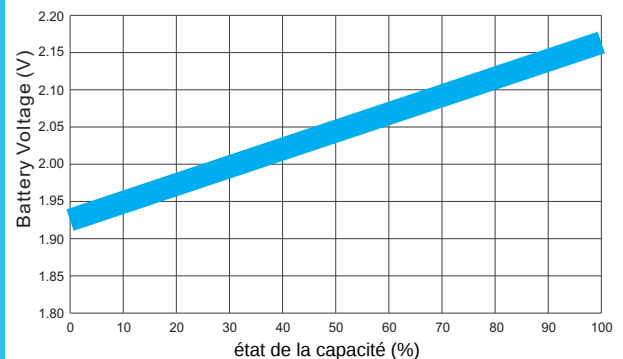
Relation entre OCV et état de charge(20°C)
