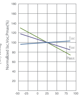
Influence de la température (Isc, Voc, Pmax)
